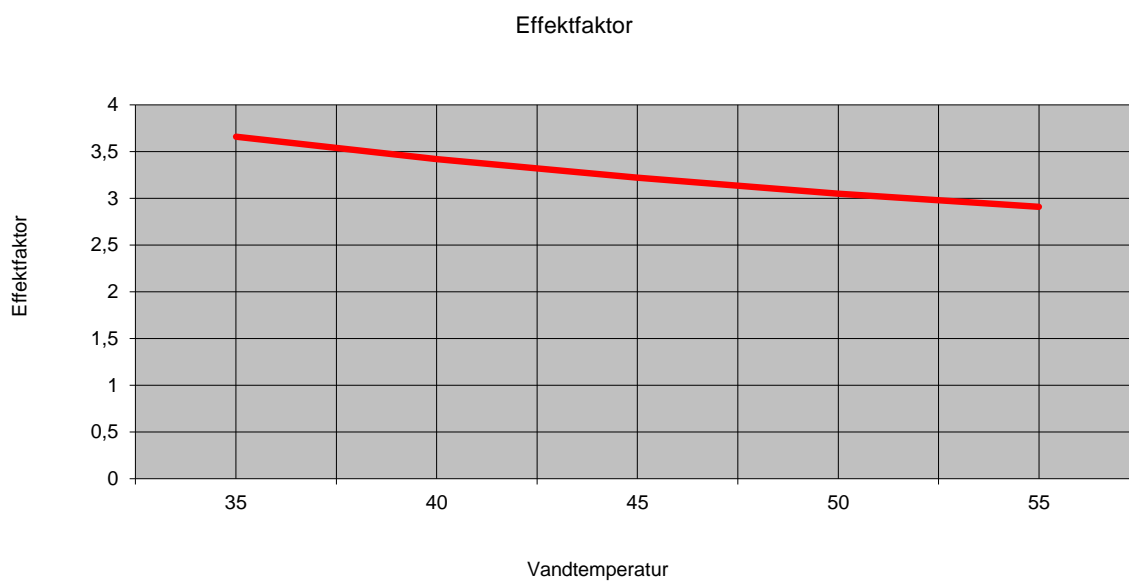
Figur 6: Effektfaktor
