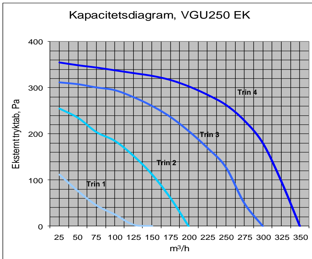
Figur 4: Kapacitetsdiagram
