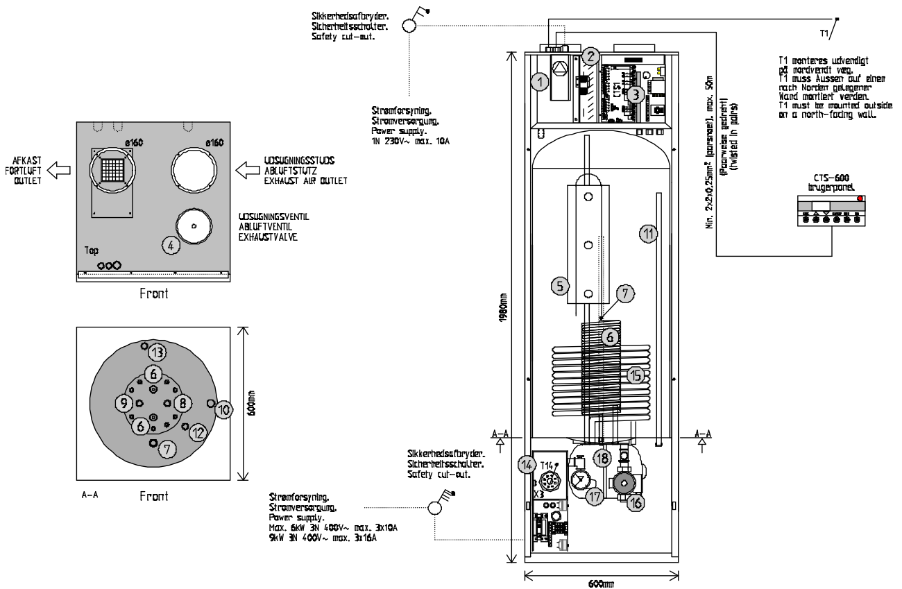
Figur 1: Principtegning
